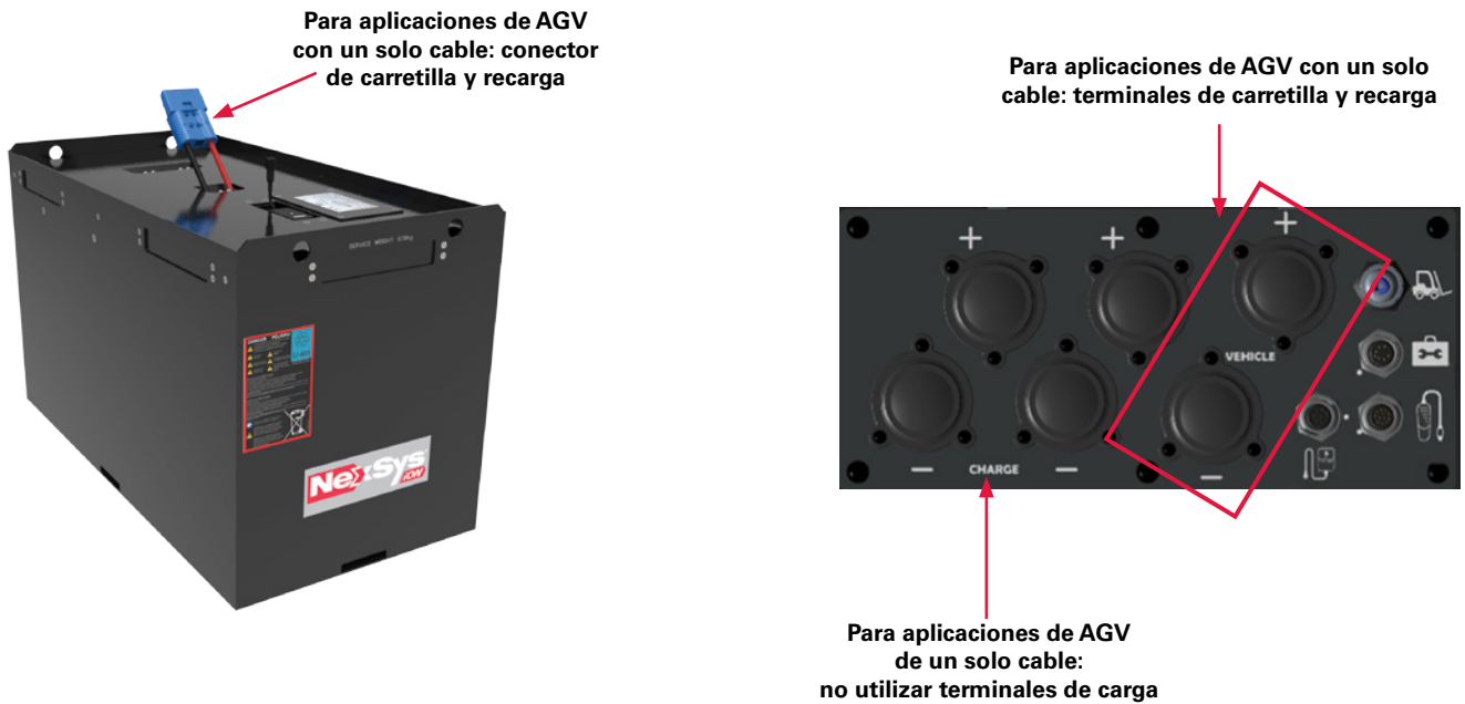
Figura 4: Aplicaciones de AGV con un solo cable
