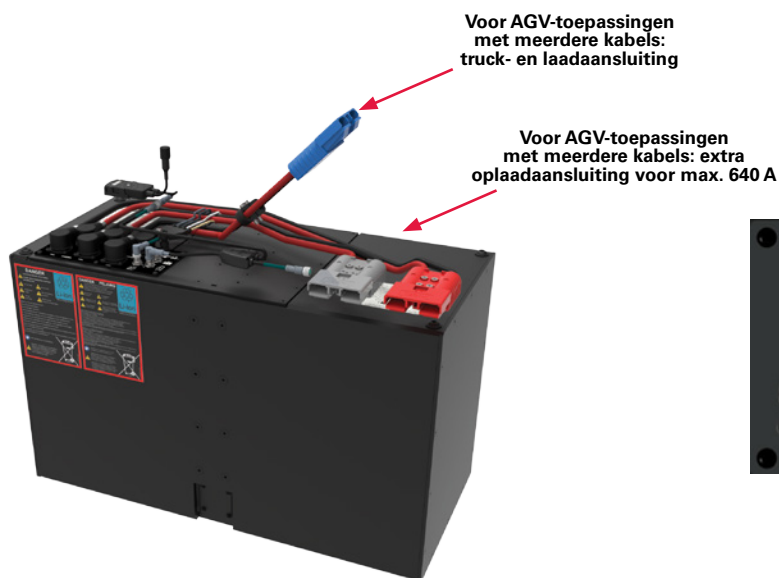
Afbeelding 5: AGV-toepassing met meerdere kabels
