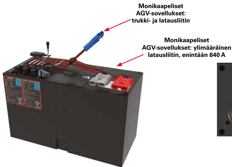
Kuva 5: Monikaapelinen AGV-sovellus
